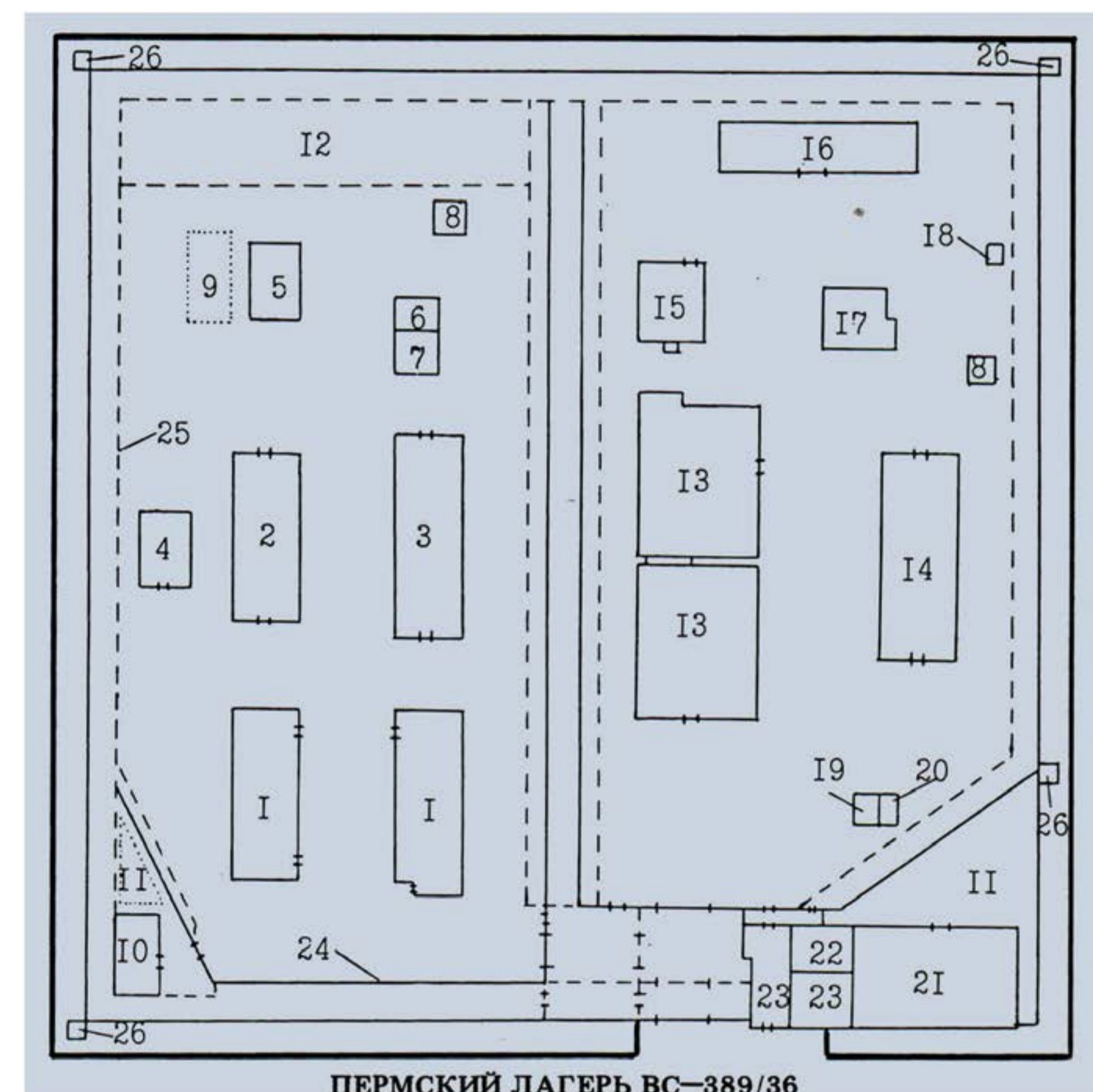
Карта-схема ИТК-35 (ст. Всесвятская Свердловской ж.д.)
